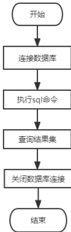
图 5-6 嵌入式 SQL-C 程序开发流程
