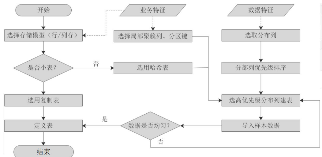
图 6-2 表定义流程
