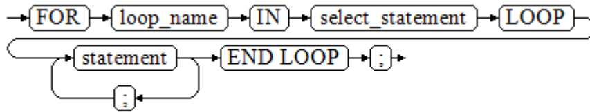
图 10-43 FOR_AS_loop::=
